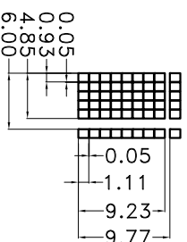
SCALE 1:2
